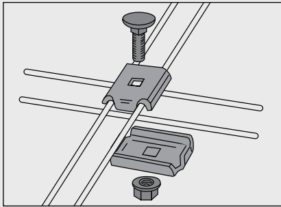
Till en skarv i botten av stegen åtgår: 2 st Beslag B2 1 st Skruvsats B13.
