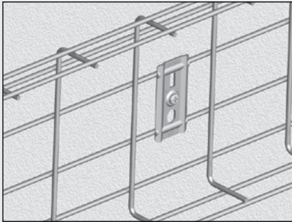
Beslag B1 kan användas som väggfäste för att montera trådstege på vägg.
