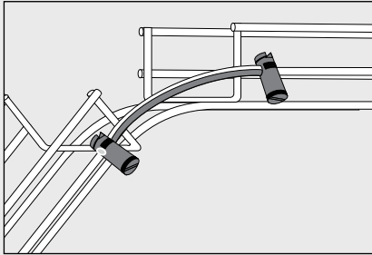
Jordkabelfästet monteras för att säkra potentialutjämningen.
