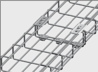
Skarvning av två C-trådstegar 220x80.
