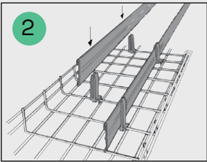
Skiljeplåten B36 snäppmonteras i plåthållaren.
