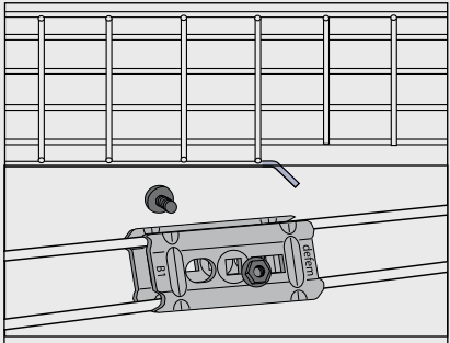
För att erhålla ett kabelvän-ligare innerhörn kan 2 st Beslag B1 monteras.
