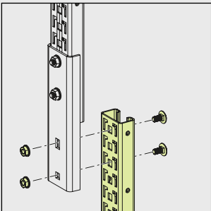
Pendelskarv 2FJ används för skarvning av Takpendel 2F och Pendel-/Ankarskena 24/48.
