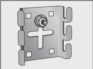
Fäste B4 eller B4 mini monteras på vägg eller golv med lämplig skruv i hörnhålen eller expander i mittenhålet.
