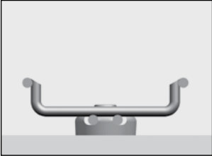
Sidovy av distansbricka B22 fäst till minitrådstege B30-U.
