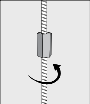
Skarvmutter B42 används för skarvning av två pendlar. Skruva fast skarvmuttern på den övre stängen till mitten av muttern. Skruva sedan i den undre pendeln i skarvmuttern. Drag åt.
