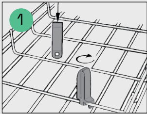
Plåthållaren vrids enkelt fast på stegens bottenråd.
