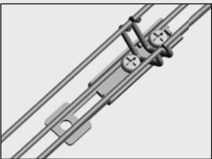
Skarvning av två Trådstegar Mini B30-D med Skarvfäste B20.
