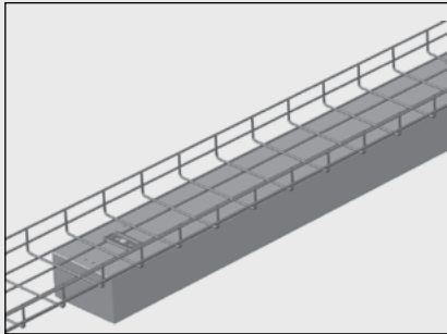
Beslag B1 kan monteras över mittentrådarna på trådstegar, alla bredder, som bärare av t ex armaturer.
