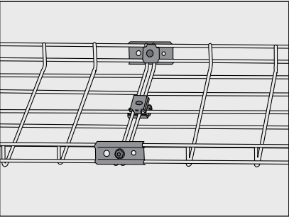
Trådstege 320 skarvas med: 2 st Beslag B1 4 st Beslag B2 3 st Skruvsats B13.
