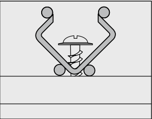
Kan monteras med skruv med stor skalle, lämplig för trä, betong etc.
