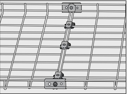
Trådstege 522 och 622 skarvas med: 2 st Beslag B1 8 st Beslag B2 5 st Skruvsats B13.
