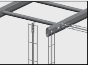
Skarvfästet kan användas för vertikal och horisontell montering av Minitrådstegar på trådstegar och kabelstegar.
