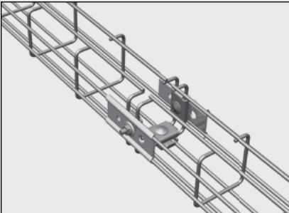
Skarvning av två C-trådstegar 75x75.
