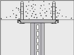
Monteras i tak med Expander eller betongskruv.
