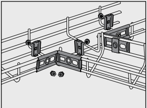
För att montera avgrening med önskad vinkel används: 2 st Vinkelbeslag B27 4 st Beslag B2 4 st Skruvsats B13.
