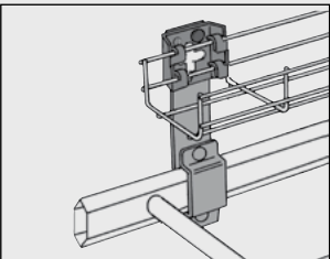
Trådstege 53 och 75 monteras på Kombi-beslag B21 med Fäste B4 mini och 2 st Skruvsats B13.
