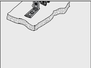
Kan användas som ändfäste mot tak eller golv, monteras med: 2 st Vinkelbeslag B27 2 st Beslag B2 2 st Skruvsats B13.
