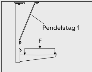
Utböjning av Takpendel 2FB minskas genom att montera Pendelstag 1 alt P/A-skena och Stagfäste 60/40. Belastning enligt nedanstående tabell.
