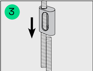
3. För ner Ovalmuttern över pendlarna som nu blir låsta.
