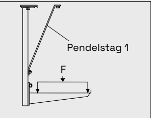
Utböjning av Takpendel 2F minskas genom att montera Pendelstag 1 alt P/A-skena och Stag-fäste 60/40. Belastning enligt nedanstående tabell.
