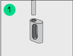
1. Ovalmutter B50 används för skarvning av pendlar. För in den övre stängen i muttern till önskat läge.
