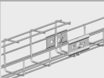
Beslag B1 och B2 används vid skarvning av trådstegar. Exemplet visar en G-tråd- stege skarvad med en standardtråd- stege.
