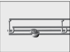
Montering av steg B30-D med Distansbricka B22.
