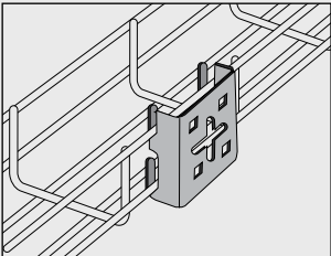
Trådstegen kan även monteras horisontellt med botten mot väggen eller mot gavel.
