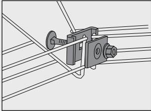
Horontella avvinklingar skarvas med Beslag B3.
