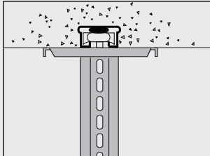
På Ingjutningsskena monteras Takpendel 2FB med T-skruv.
