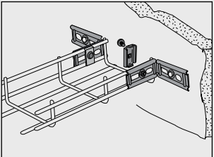
Kan användas som ändfäste mot vägg, monteras med: 2 st Vinkelbeslag B27 2 st Beslag B2 2 st Skruvsats B13.
