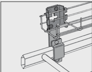
Trådstege 120 monteras på Kombibeslag B21 med Fäste B4 och 2 st Skruvsats B13.
