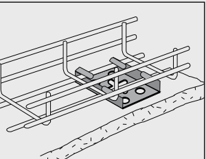
Trådstegen kan även monteras vertikalt med botten mot golv.
