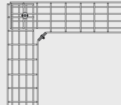
Trådstege 53 till 220 skarvas med: 2 st Beslag B1 2 st Beslag B2 2 st Skruvsats B13.
