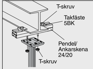
På balkar i tak monteras Takpendel 2FB enligt ovanstående figur. Då balkens flänstjocklek är max 13 mm används Takfäste 5BK-10 och T-skruv 26U/40. Vid flänstjocklek max 30 mm används Takfäste 5BK-30 och T-skruv 26U/50.
