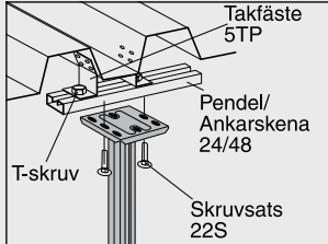
I plåttak med trapetsprofile-rad plåt monteras Takpendel 2FB enligt ovanstående figur.
