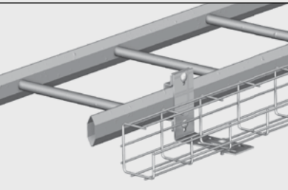
Montering mot kabel-stege med Kombi- beslag B21 90°.
