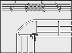
Trådstege 75 vinklas till rundad 90° vinkel genom att markerade trådar klipps bort, tråden böjs och innerhörnet skarvas med 1 st Beslag B3.
