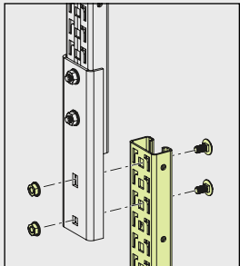
Pendelskarv 2FJ används för skarvning av Takpendel 2FB och Pendel-/Ankarskena 24/48.
