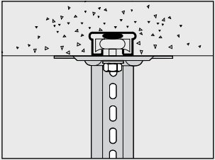
På Ingjutningsskena monteras Takpendel 2F med T-skruv.
