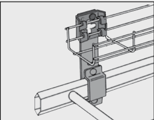
För montage av Trådstege på Kombi-beslag 21 används Fäste B4 eller B4 mini.
