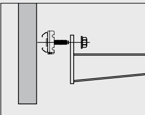
Konsol 50 med T-skruv.
