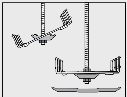
Montera Bärokets undre del för 320-422 efter att stegen applicerats i den övre delen. 2 st Skruvsats B13 används.
