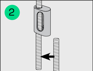
2. Lägg den undre stängen mot den övre så att gängorna griper in i varandra.
