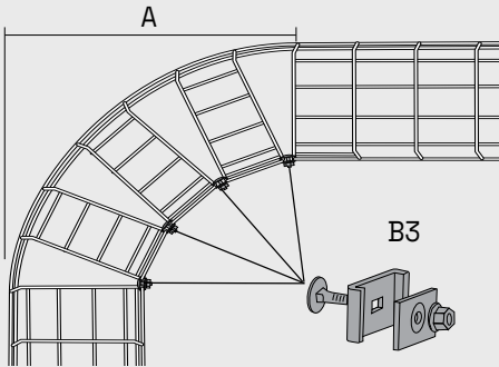
Trådstege 120 till 622 vinklas till rak 90° vinkel genom att varannan markerad sektion klipps bort, tråden böjs och innerhörnet skarvas med Beslag B3 enligt tabellen.
