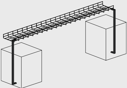
Lång dubbelanslutning - i bästa fall EMC-neutral
