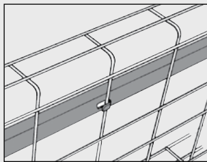
Avskiljningsplåtens montageflikar underlättar fastsättningen. Flikarna nyps fast runt bottentråden.
