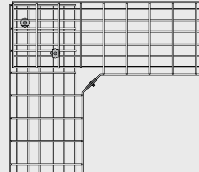
Trådstege 320 till 422 skarvas med: 2 st Beslag B1 4 st Beslag B2 3 st Skruvsats B13.
