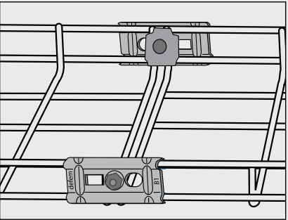
Trådstege 53 till 220 skarvas med: 2 st Beslag B1 2 st Beslag B2 2 st Skruvsats B13
