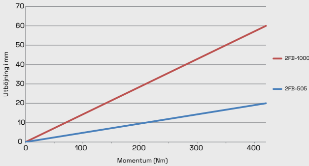
Utböjning av Takpendel 2FB minskas genom att montera Pendelstag 1 alt P/A-skena och Stagfäste 60/40. Belastning enligt nedanstående tabell.
