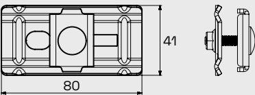
Montera Skarv B52 över stegskarven.
