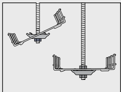
Bärok B39/120-220. Vinkla in Trådstegen i Bärokets övre del och kläm fast flikarna.
