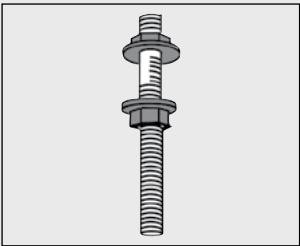
Flänsmutter B43 monterats på Pendel B41 och W76 för att låsa bärok och takfästen.
