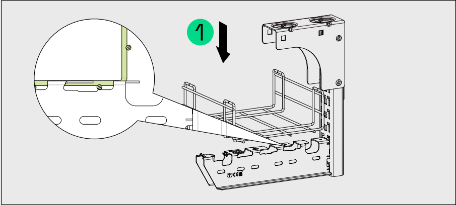
1. Placera de långsgående trådarna i konsolens spår enligt bild ovan.
