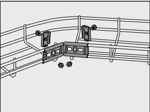
Vinkeln justeras med vinkelbeslaget till önskat gradtal.
