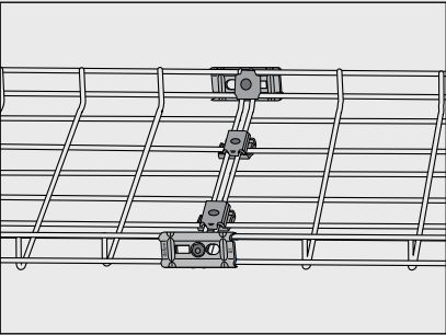
Trådstege 422 skarvas med: 2 st Beslag B1 6 st Beslag B2 4 st Skruvsats B13.
