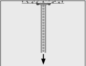
Tillåten belastning för Takpendel 2F (Tp) vid symmetrisk belastning = 1353 kg.
