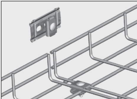
Montera Skarv B52 över stegskarven.
