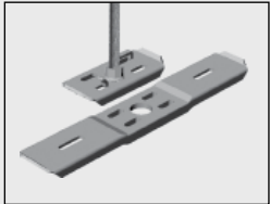
Pendel B41 och W76 monterats till Bärok B39 med 2 st Flänsmutter B43.
