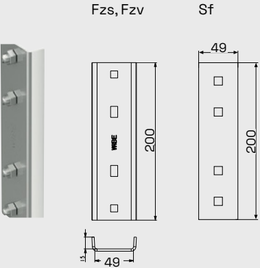
Pendelskarv 2FJ
