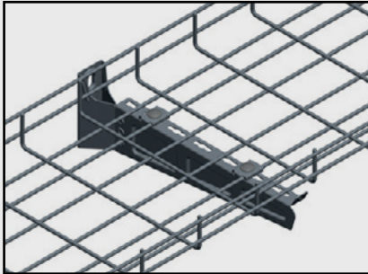
Trådstege monteras med 2 st Beslag B2 och 2 st Skruvsats B13 på Konsol 50i.
