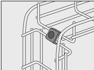
Vertikal avvinkling skarvas med 1 eller flera Beslag B3 beroende på stegbredden.
