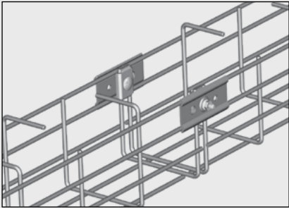
Skarvning av Z-trådstege med Beslag B1/B2.
