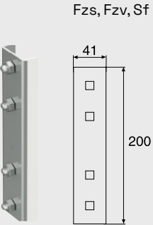
Pendelskarv 2J
