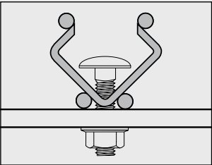
Kan monteras med Skruvsats B13.
