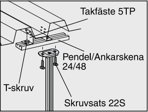
I plåttak med trapets-profilerad plåt monteras Takpendel 2F enligt ovanstående figur.
