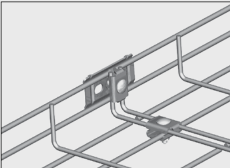
Skruva åt skruven och skarvningen är klar.
