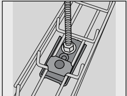
Till Trådstege 53 och 75 kan Beslag B1 användas som bärok. Monteras med 1 st Beslag B2, 1 st Skruvsats B13 och 2 st Flänsmutter B43.
