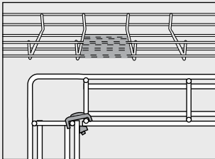
Trådstege 53 vinklas till rak 90° vinkel genom att markerade trådar klipps bort, tråden böjs och innerhörnet skarvas med 1 st Beslag B3.
