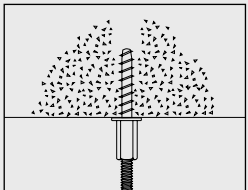
Takmontage, pendel med Betongskruv MMS-I.
