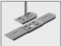
Bäroket används tillsammans med Pendel B41 och W76. Monteras med 2 st Flänsmutter B43.
