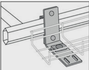
Trådstege 53, 75 och 120 monteras på Kombi-beslag B21 90° med 1 st Beslag B2 och 1 st Skruvsats B13.
