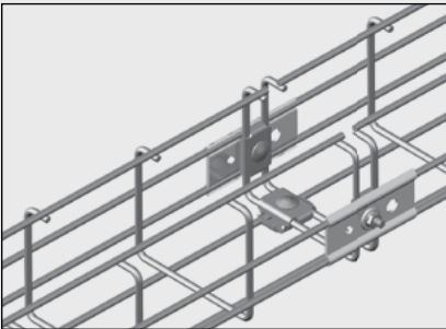
Skarvning av två C-trådstegar 120x100.
