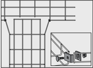
X- och T-avgreningar skarvas med Beslag B3.
