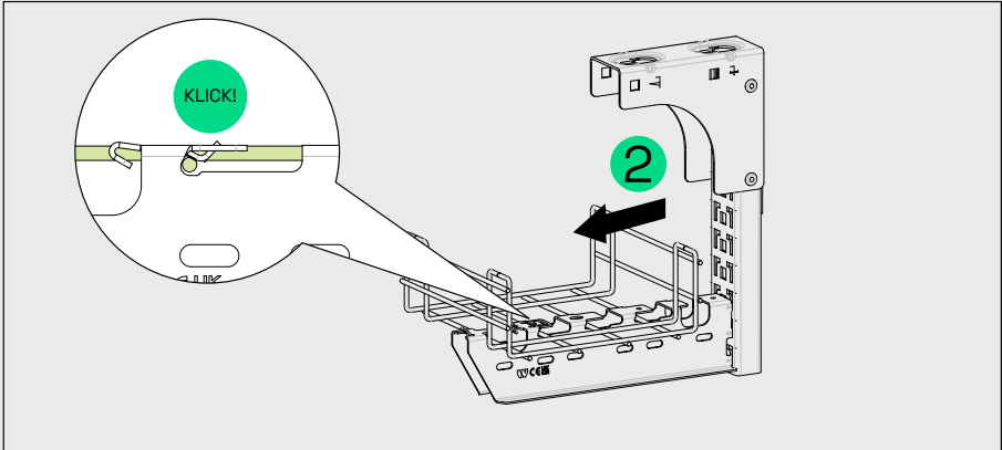
2. Dra trådstegen horisontellt mot konsolens spets tills tråden passerar låsfliken och hamnar i rätt läge med ett klick.
