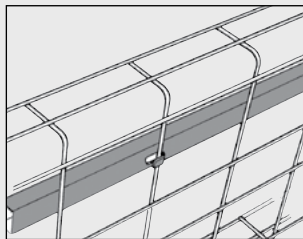
Telerännans montageflikar underlättar fastsättningen. Flikarna nyps fast runt bottentråden.
