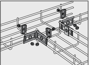
För att montera 90° T-avgrening används: 2 st Vinkelbeslag B27 4 st Beslag B2 4 st Skruvsats B13.
