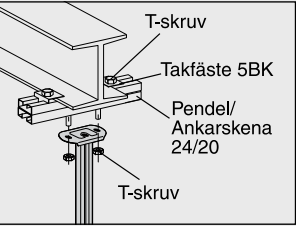
På balkar i tak monteras Takpendel 2F enligt ovanstående figur. Då balkens flänstjocklek är max 13 mm används Takfäste 5BK-10 och T-skruv 26U/40. Vid flänstjocklek max 30 mm används Takfäste 5BK-30 och T-skruv 26U/50.
