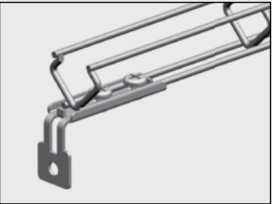
Kan användas både för skarvning och som ändfäste mot golv, vägg och tak.
