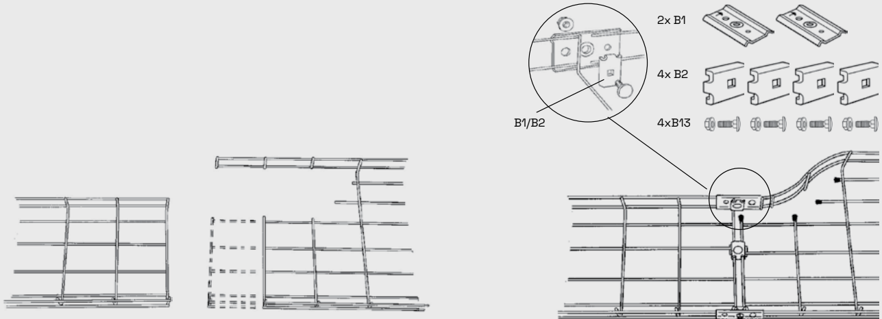
Ensidig övergångsskarv / B1, B2, B13 alt B52
