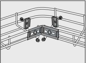
För att skarva vinkeln används: 1 st Vinkelbeslag B27 2 st Beslag B2 2 st Skruvsats B13.
