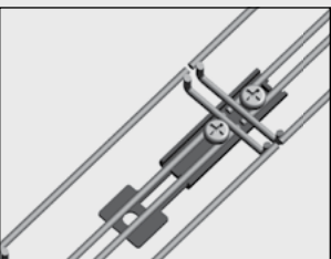
Två U-stegar skarvade med Skarvfäste B20.
