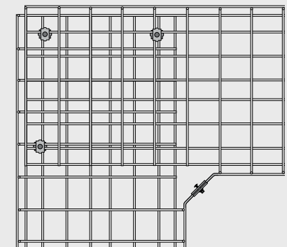
Trådstege 522 till 622 skarvas med: 2 st Beslag B1 6 st Beslag B2 4 st Skruvsats B13.
