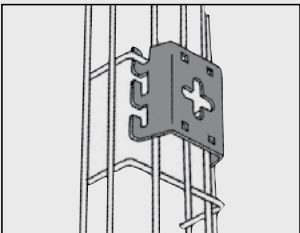
Trådstegen kan även monteras vertikalt med botten mot väggen.
