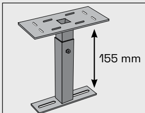
Stödbenet är justerbart i höjd från 215 till 370 mm.
