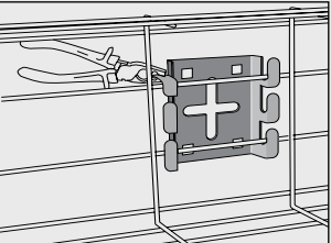
För säkrare montage bör flikarna på fästet vikas runt stegens tråd med en tång.
