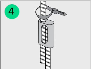
4. Drag åt ett buntband över ovalmuttern som låsning.
