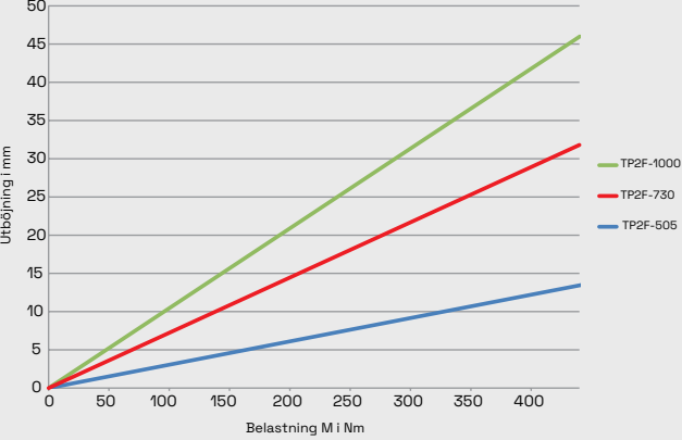
Vid värden utanför diagrammet kontakta Wibe
