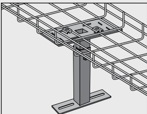
Trådstegen monteras på stödbenet med lämpligt antal Beslag B2.
