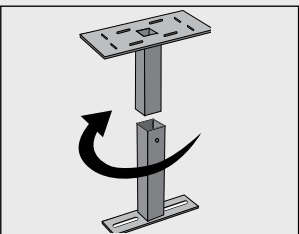
Över eller underdel kan vridas 90° och hopmonteras.
