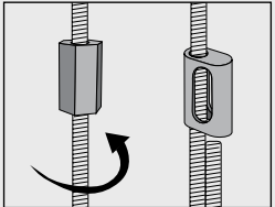
Pendeln kan skarvas med Skarvmutter B42 eller Ovalmutter B50.
